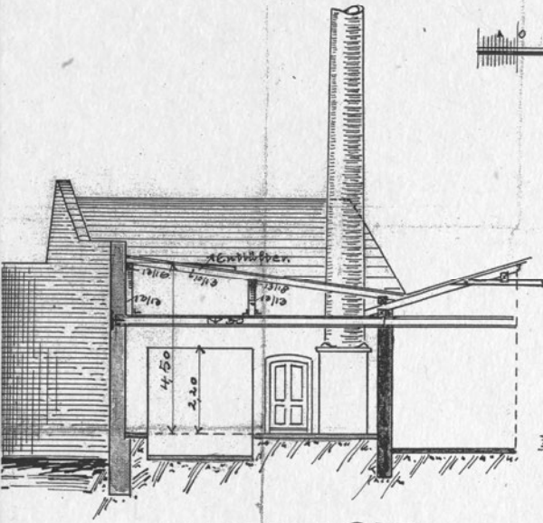
- SCHNITT C-D -
