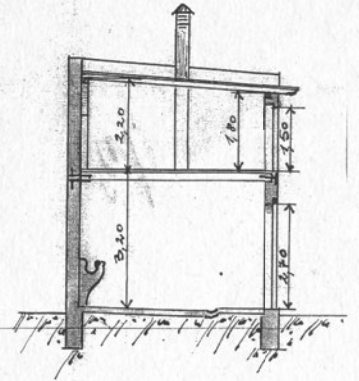
- SCHNITT E-F -
